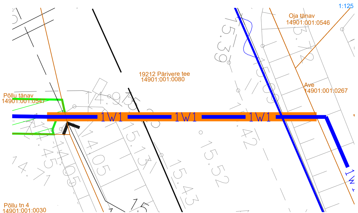
Ristmävli RV-2 T 19212 teemaal km 0,2 Ø110 15 m 1250N Kinnine läbindamine
